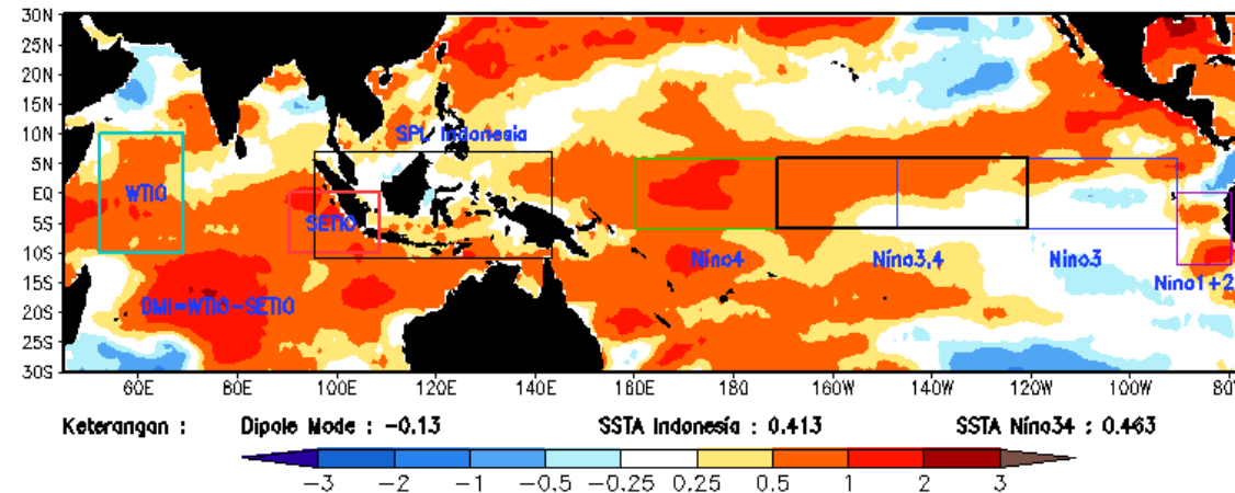
Anomali Suhu Muka Laut Maret 2020
