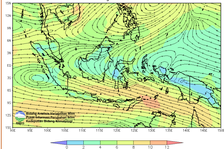
Prakiraan Angin 850mb 202010
