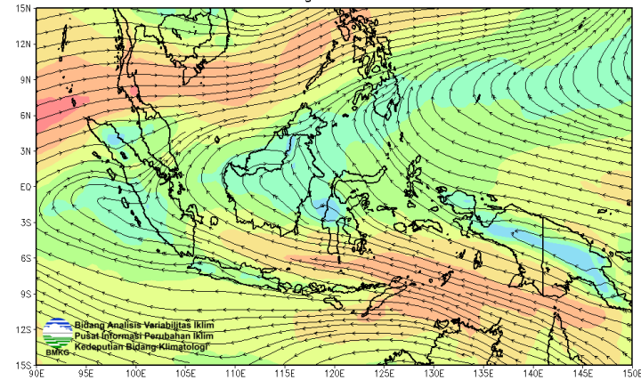
Prakiraan Angin 850mb 202010
