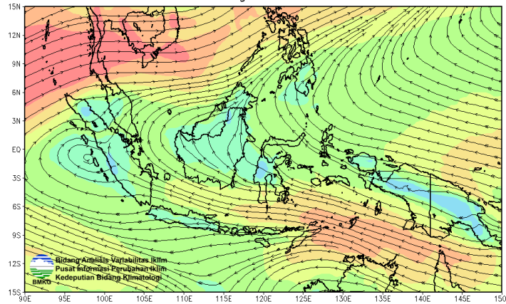
Prakiraan Angin 850mb 202008
